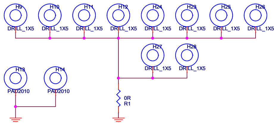
液晶框固定孔
